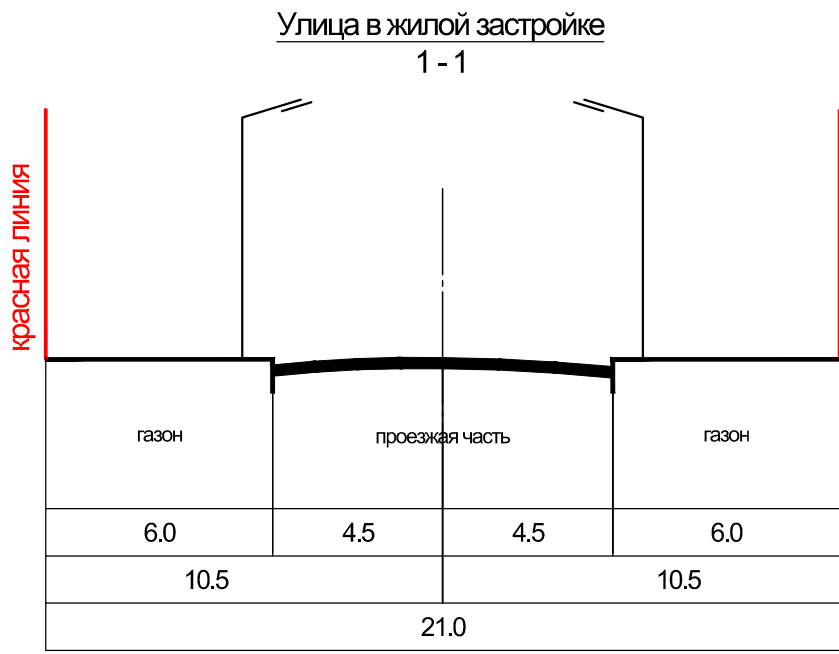
Поперечные профили улиц
