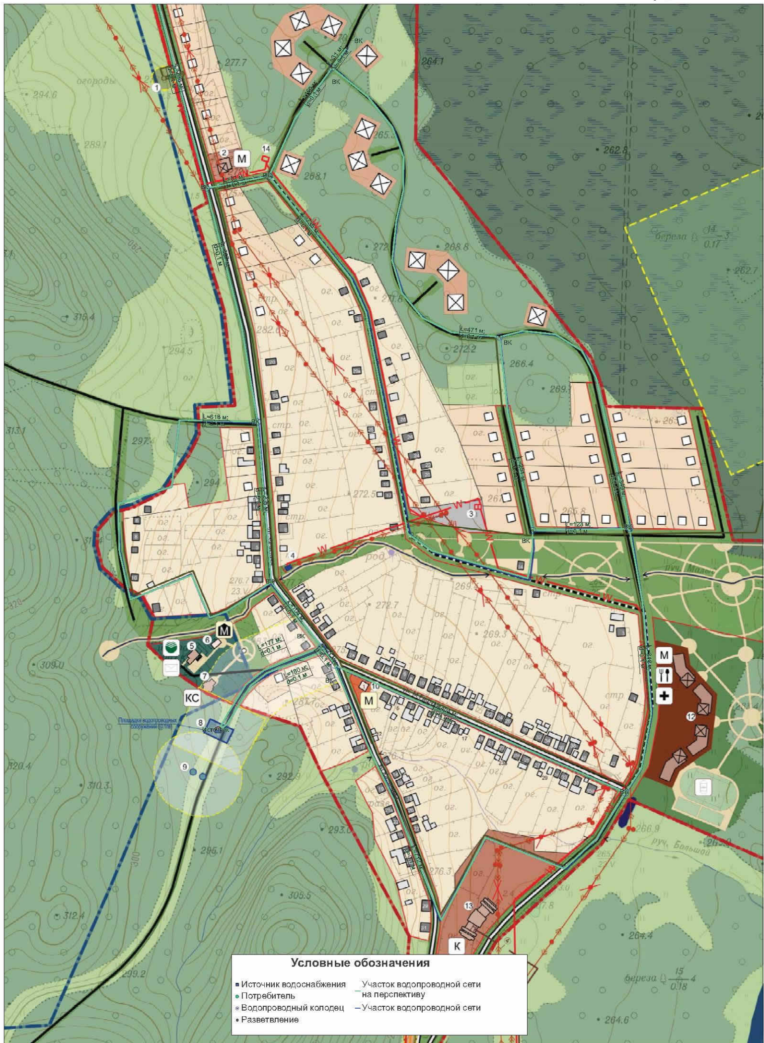
Схема водоснабжения д. Ключи
